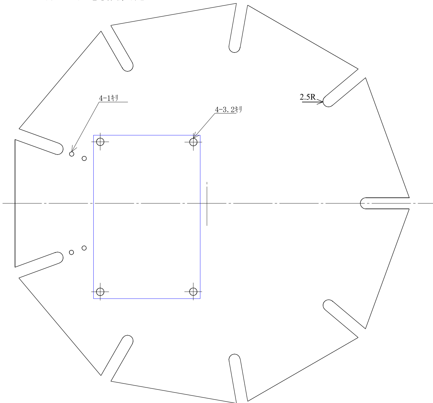
スパイダーコイル巻き枠(原寸図)
